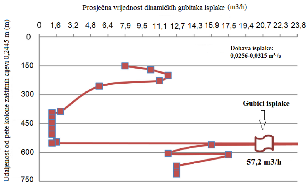
Slika 8-4. Dinamički gubici tijekom bušenja „Mud Cap“ metodom na polju u Abu Dhabiju (Al Awadhi et al., 2014)
