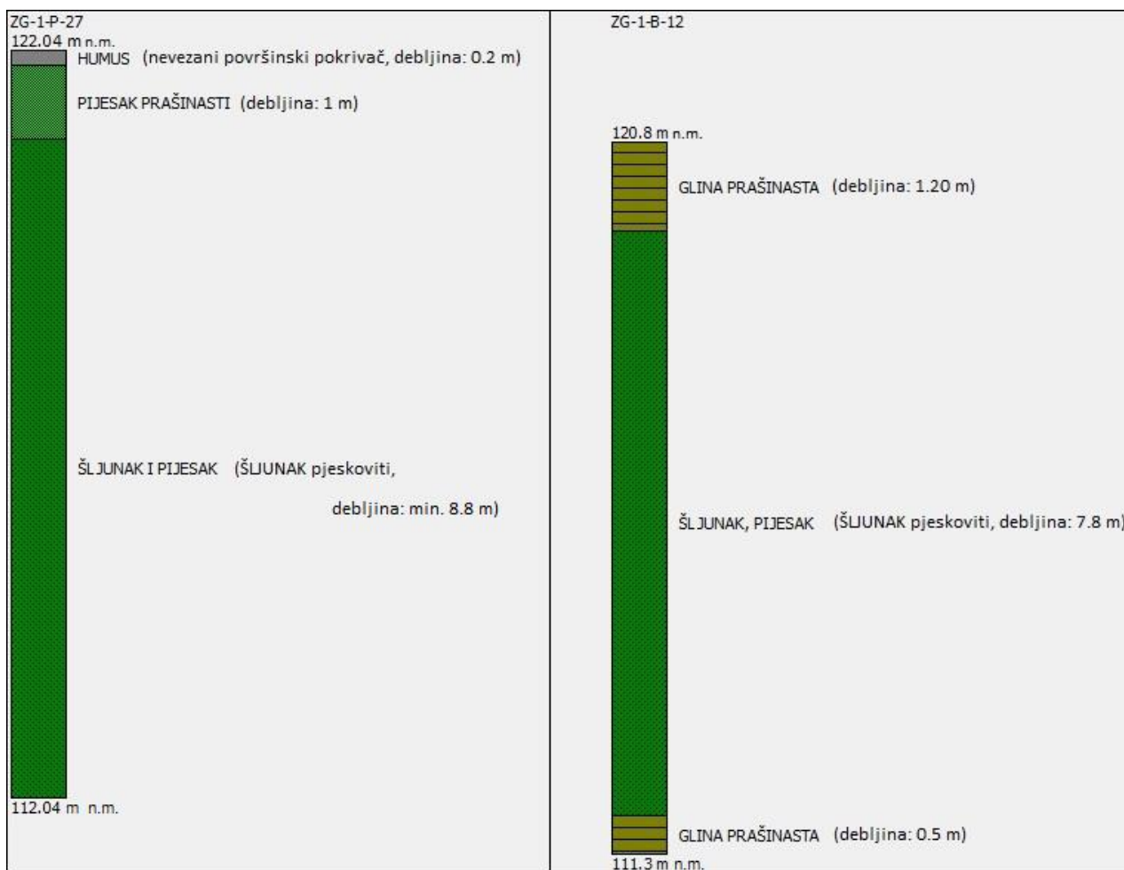
Slika 2.2 Litološki stup na području planiranog vodocrpilišta Ježdovec
