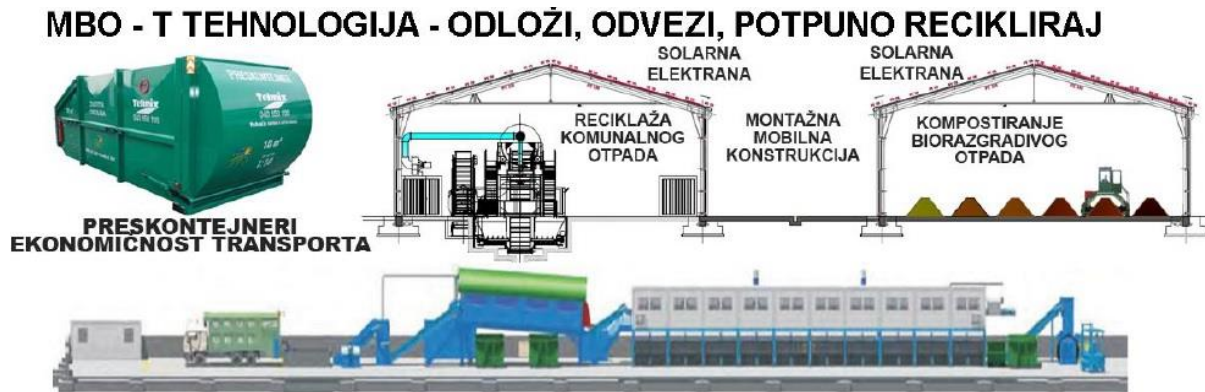
Slika 9. MBO-T tehnologija, skica pogona (izvor:www.poslovní.hr)
