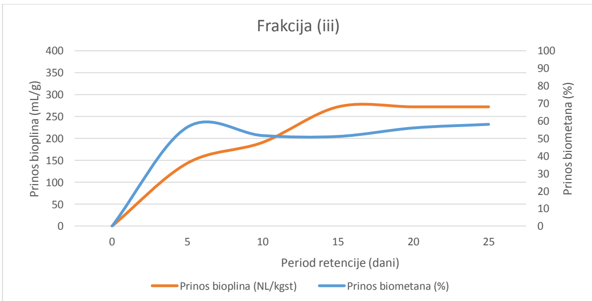
Graf 4.4.3. Krivulje proizvodnje bioplina i biometana po danima za frakciju (iii) <500 \mu\text{m}
