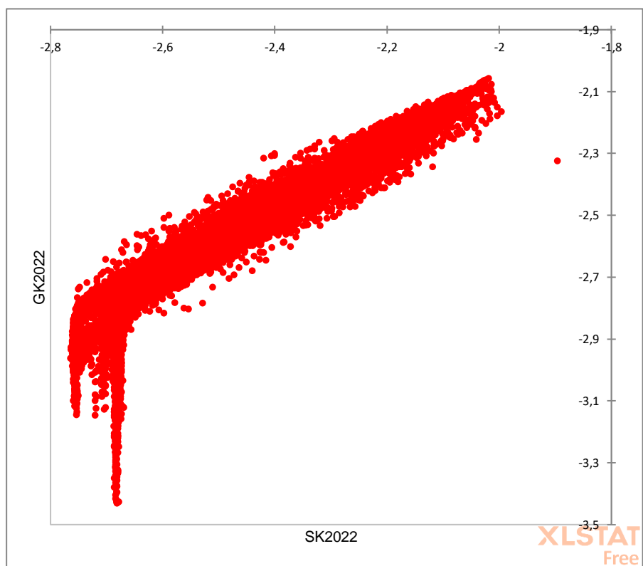
Graf 3.10. Grafički prikaz korelacija razine vodostaja glavnom i sabirnog kanala tijekom 2022. godine (izvor: autor)
