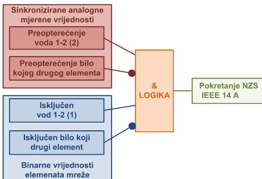
Slika 5.5 Uvjeti pokretanja NZS-e za IEEE ispitni sustav s 14 sabirnica
