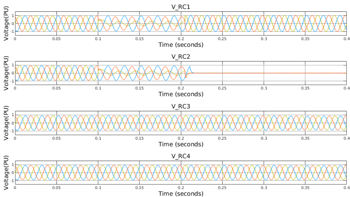
Slika 7.11: Oscillografski zapis napona RC1-RC4
