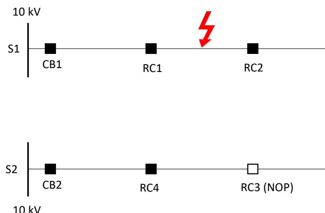
Slika 7.9: Simulacija kvara na mjestu RC1-RC2
