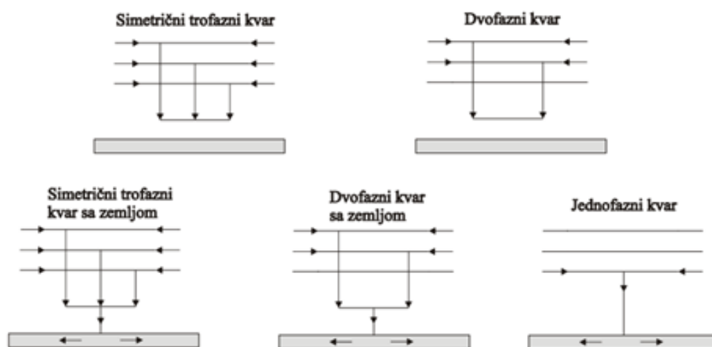
Slika 2.6: Vrste kvarova u distribuciskoj mreži
