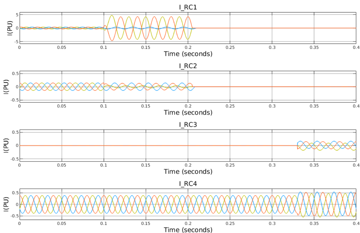
Slika 7.10: Oscillografski zapis struja RC1-RC4
