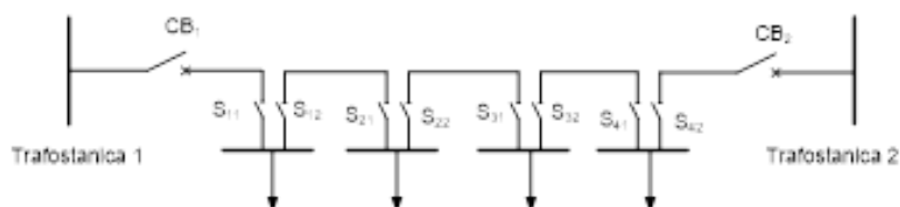
Slika 4.6: Kabela mreža bez komunikacije
