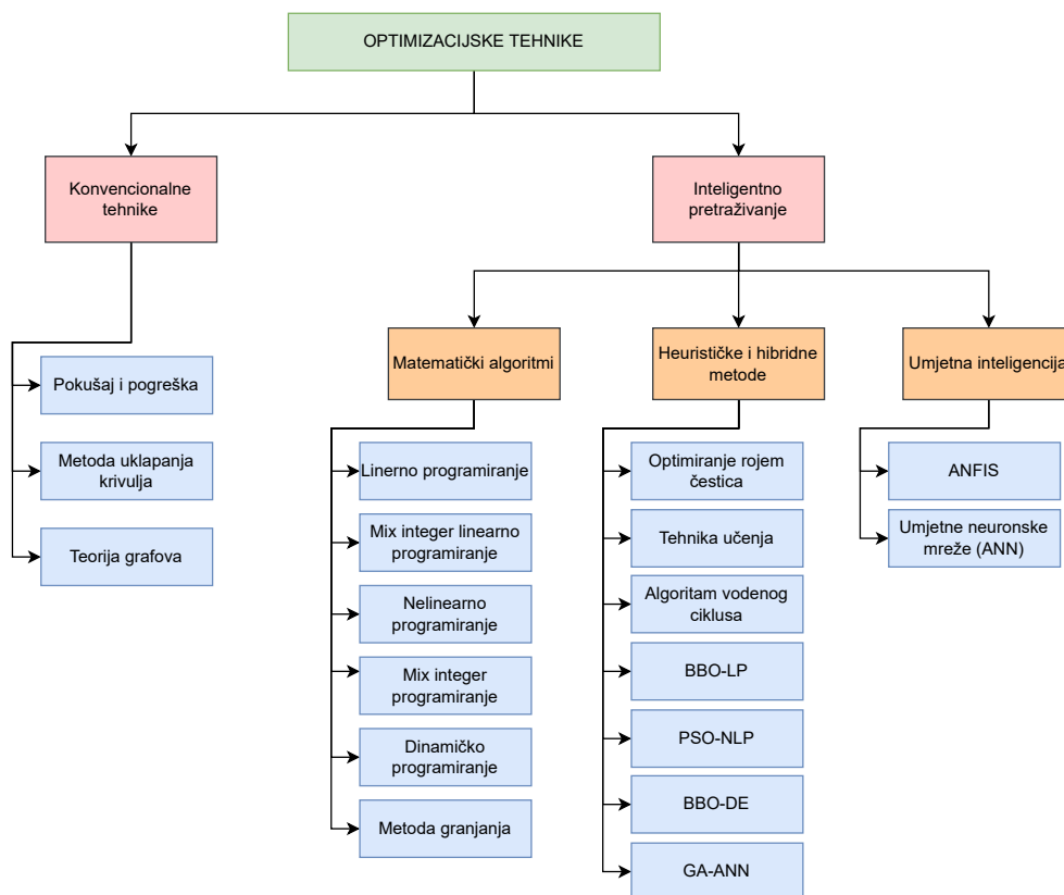
Slika 5.1: Različite tehnike i metode optimalne koordinacije nadstrujnih releja [58]
