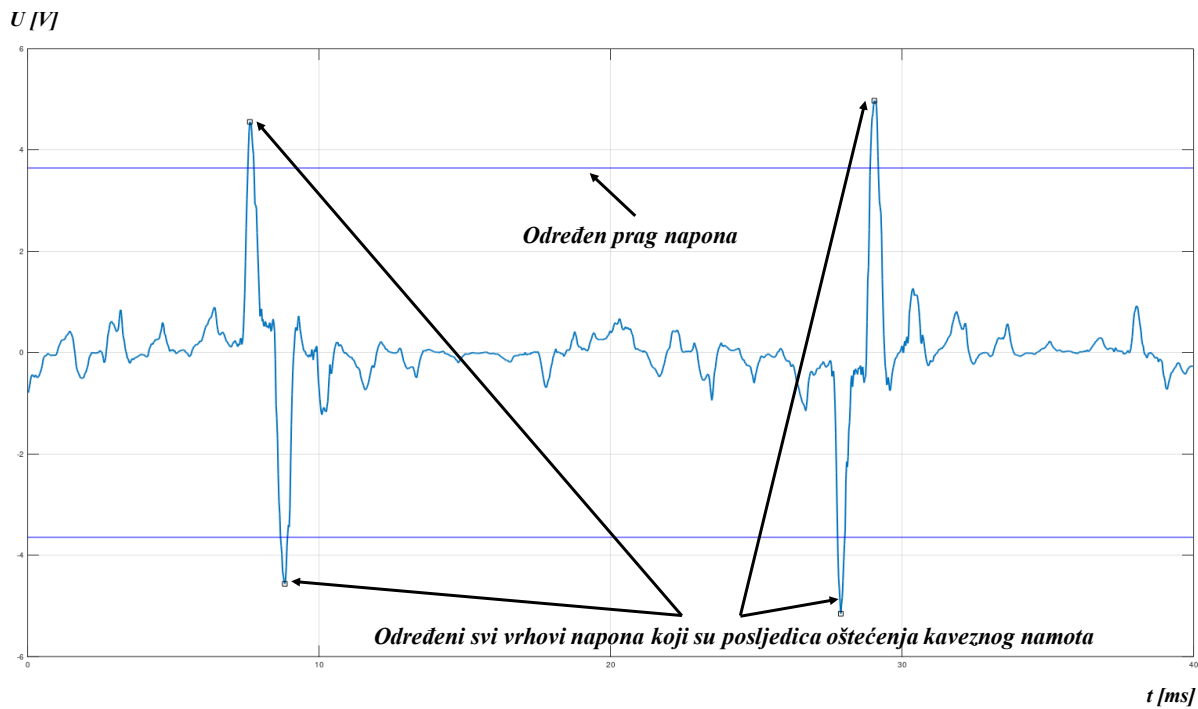
Slika 8.11 Učitani signal y – funkcijom findpeakandthreshold određen prag i vrhovi napona
