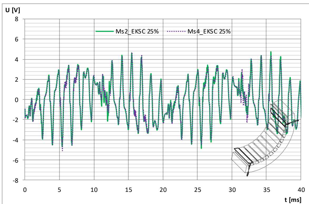
Slika 5.19 Usporedba valnih oblika induciranih napona u mjernim svicima Ms2 i Ms4 prostorno razmaknutih za 2\tau_p kod iznosa statičkog ekscentriciteta od 25 % zračnog raspora (pomak u smjeru + y osi)
