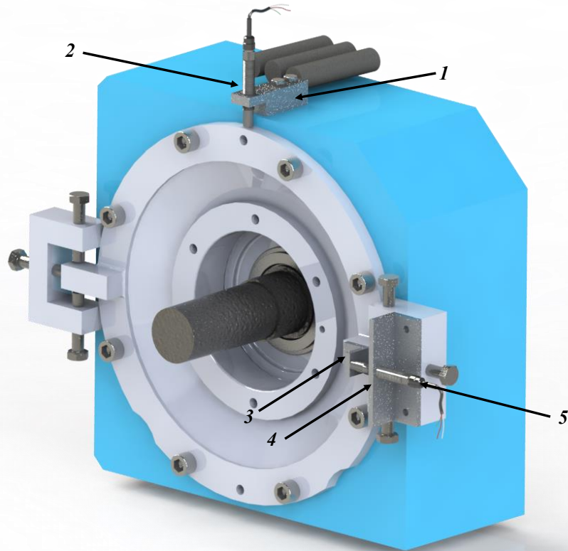
Slika 3.12 Prikaz ugradnje induktivnih senzora: 1 – nosač senzora za mjerenje u y – osi, 2 – induktivni senzor, 3 – pomoćni dio za mjerenje u x – osi, 4 – nosač senzora za mjerenje u x – osi, 5 – induktivni senzor
