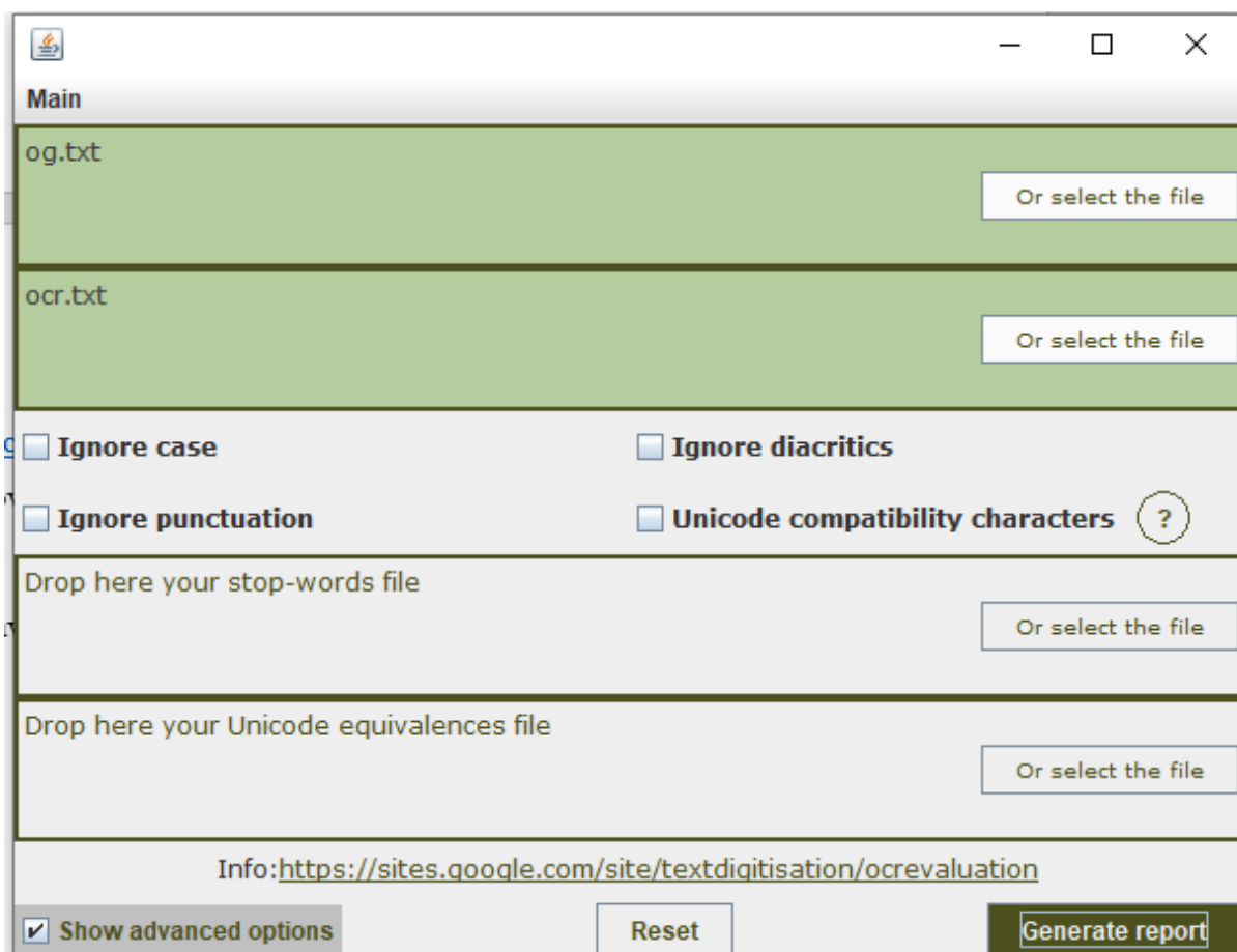
Slika 11 - OcrevalUAtion sučelje
