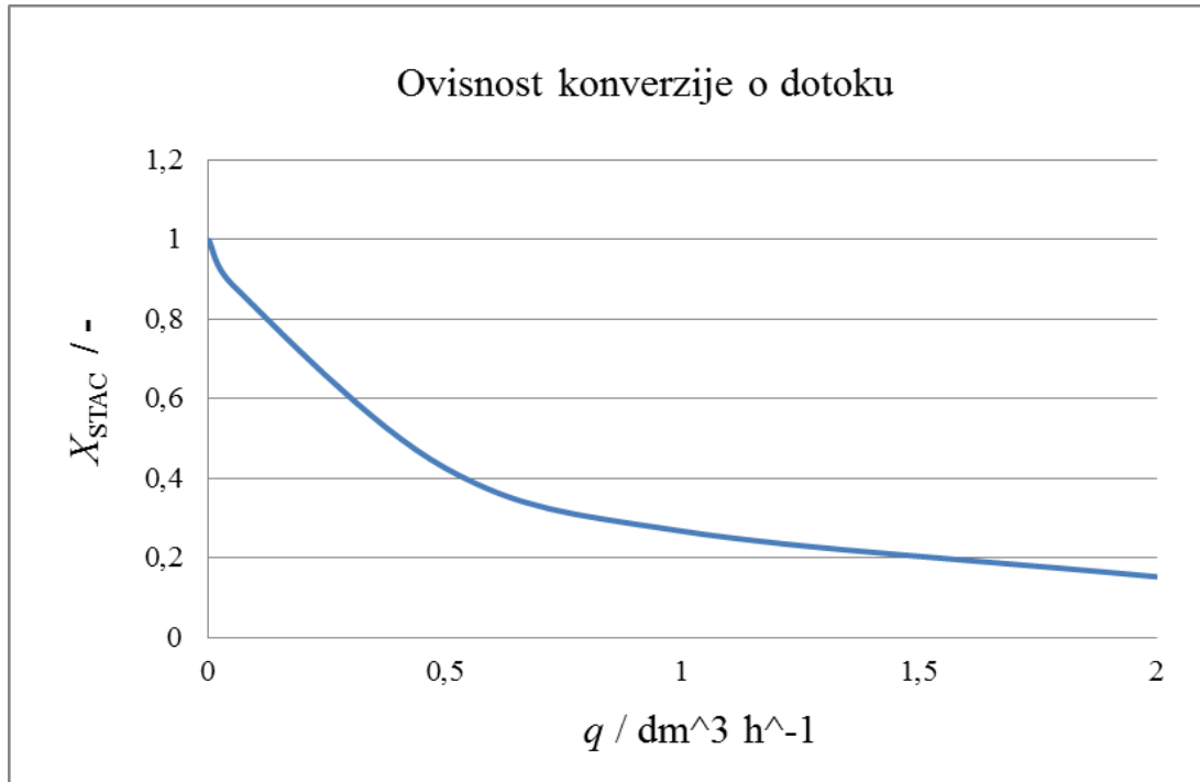
Slika 28. Grafički prikaz ovisnosti stacionarne konverzije o dotoku u reaktoru s dotokom
