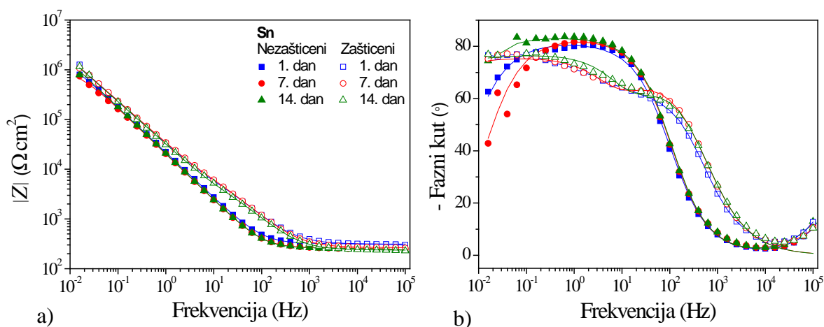
Slika 4.32. EIS – Bodeov prikaz za nezaštićeni i zaštićeni uzorak kositra prvi dan, nakon tjedan dana i nakon dva tjedna izlaganja umjetnoj kiselj kiši: a) modul impedancije i b) fazni kut (simboli – eksperimentalni podaci, linije – rezultati dobiveni korištenjem modela prikazanih na slici 4.33.). 187
