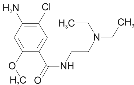
Slika 7. Struktura metoklopramida
