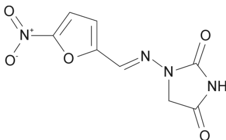
Slika 4. Struktura nitrofurantoina
