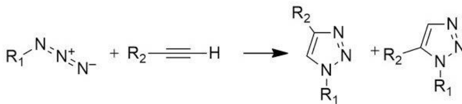
Shema 7. Huisgenova 1,3-dipolarna cikloadicija azida i alkina
