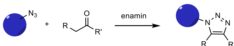
Shema 1. Huisgenova cikloadicija azida i ketona katalizirana enaminom
