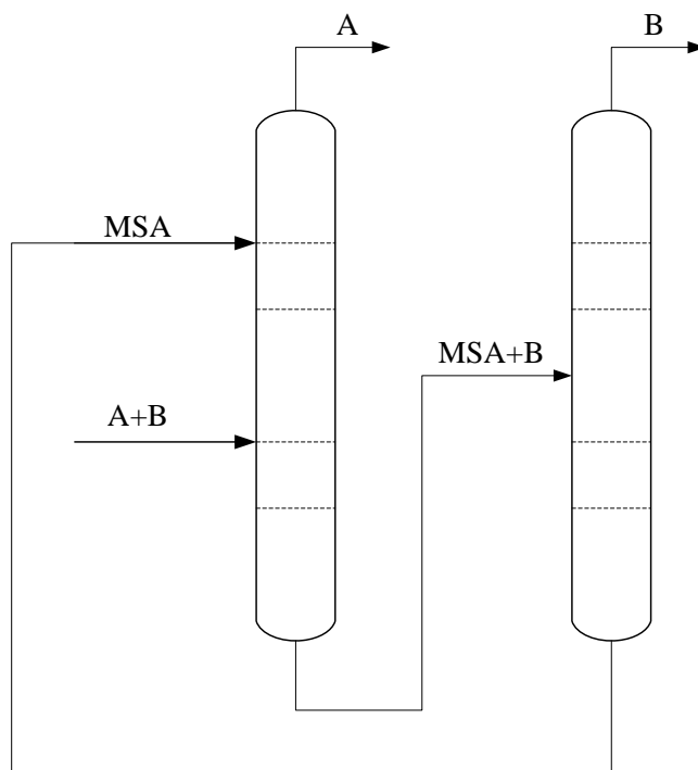
Slika 11. Shema ekstrakcijske destilacije [4].
