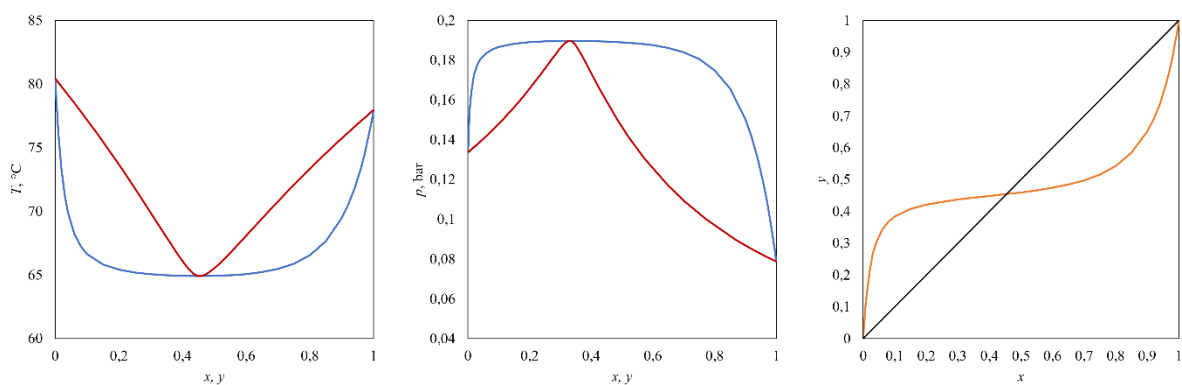
Slika 7. S lijeva na desno, T - x - y dijagram pri stalnom tlaku, p - x - y dijagram uz stalnu temperaturu te x - y dijagram) za azeotropne sustave s minimalnim vrelištem.
