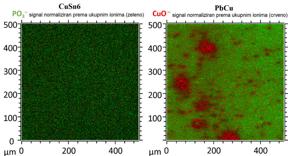
Slika 4.37. ToF-SIMS prikaz negativnih iona koji predstavlja raspodjelu 16-fosfonoheksadekanske kiseline (signal PO_3^- ) i bakrenih oksida (signal CuO^- ) za a) CuSn6 i b) kvaternarnu bronzcu. 187
