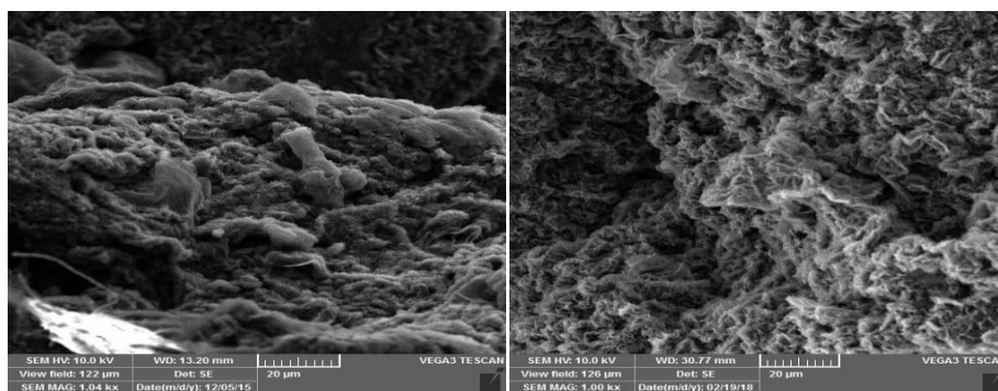
Slika 4.15 SEM uzoraka h-rGO-0 i h-rGO-PANI-0.
