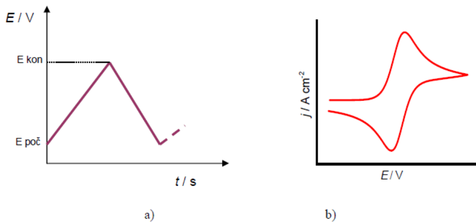
Slika 2.14 Signal a) pobude i b) odziva u cikličkoj voltametriji.
