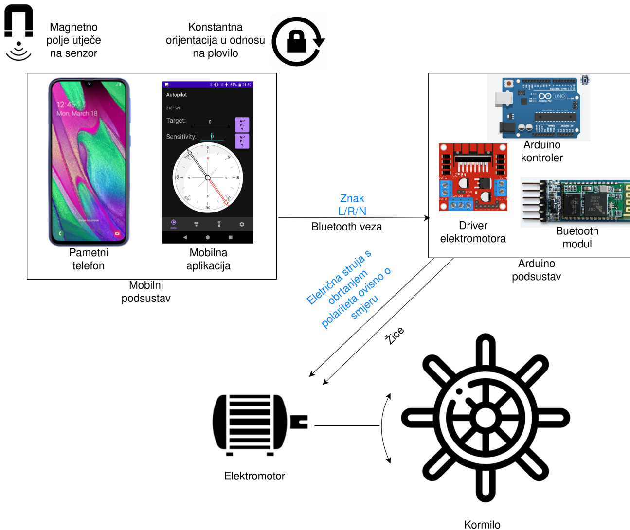
Slika 27 Arhitektura implementiranog rješenja autopilota
