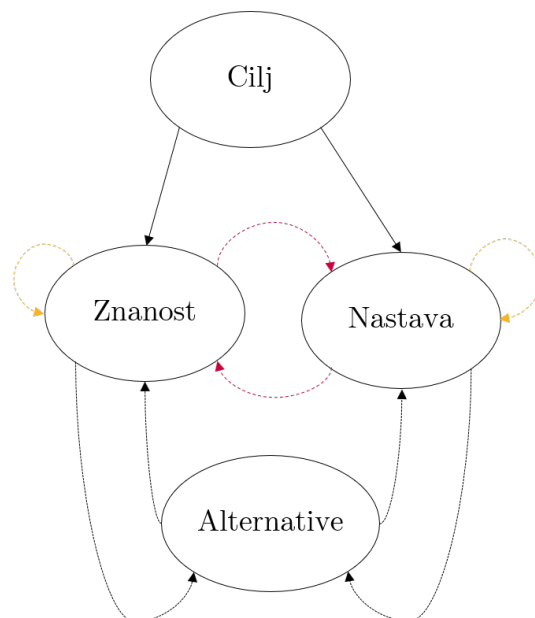
Slika 3.7: Struktura problema odlučivanja, razina klastera
