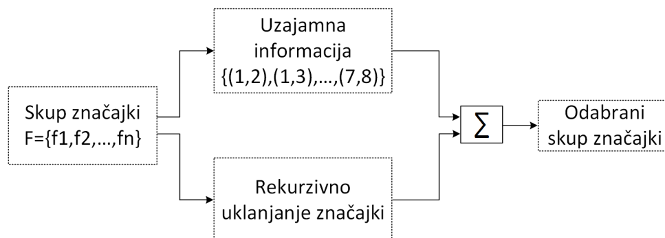
Slika 4.10: Proces smanjenja broja značajki
