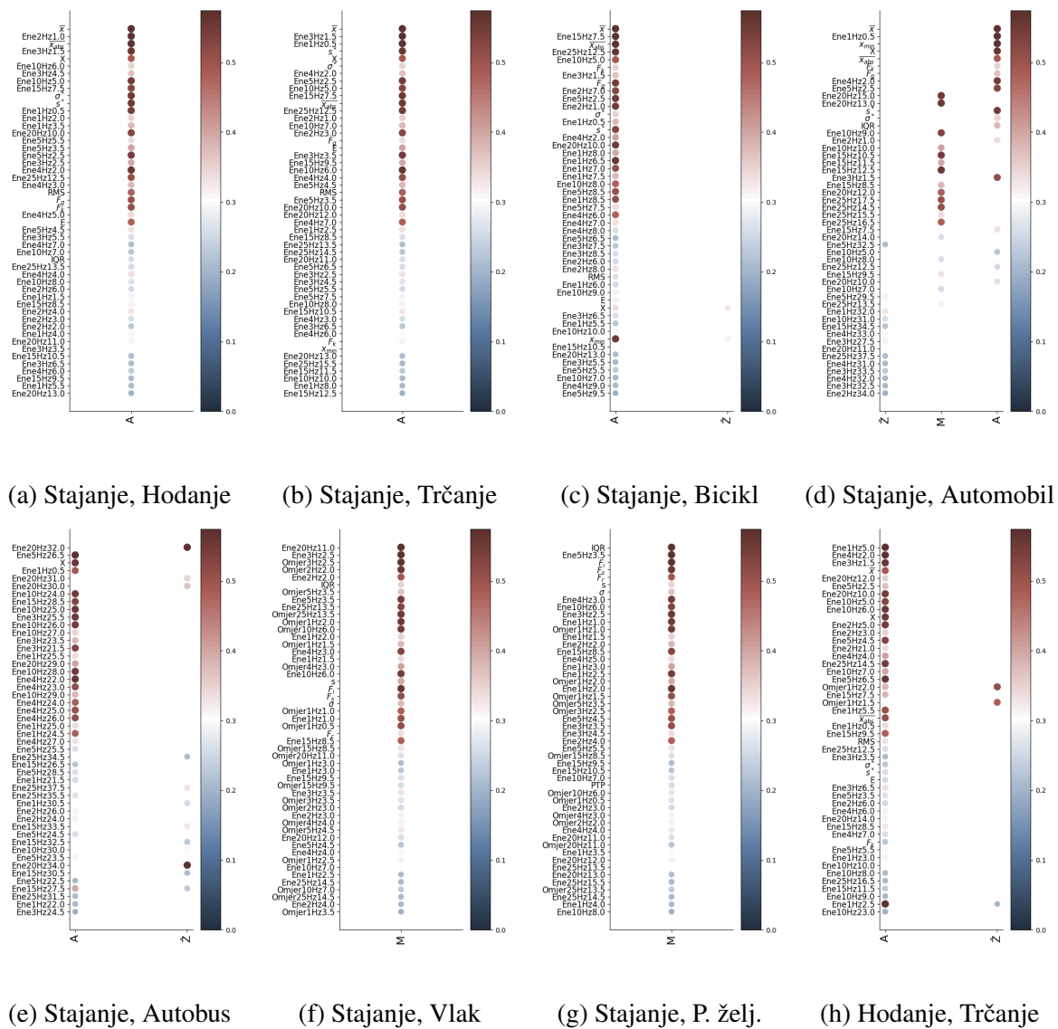
Slika 4.23: MI vrijednost za svaki par modova prijevoza uključenih u klasifikaciju
