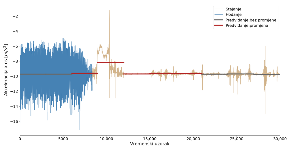
Slika 4.18: Vrijednost sirovih podataka u trajektoriji po x osi akcelerometra i srednja vrijednost akceleracije
