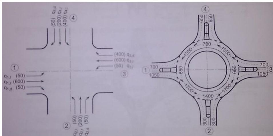
Slika 19. Pretvorba brojnog prometa na klasičnom raskrižju u kružno
