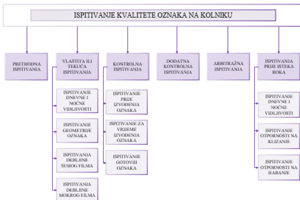
Slika 35. Vrste ispitivanja kvalitete oznaka na kolniku
