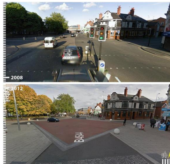
Slika 36. Spared space koncept u zoni raskrižja
