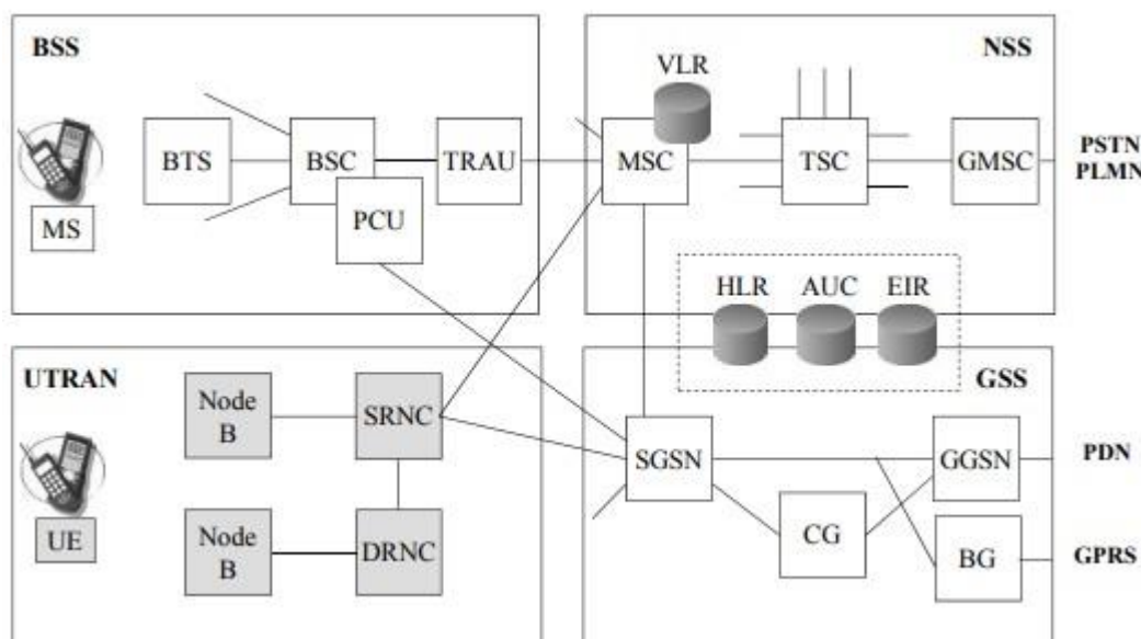
Slika 5. UMTS arhitektura [1]
