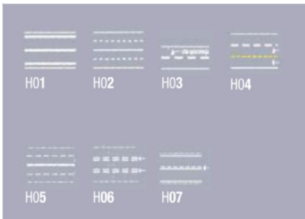
Slika 6. Primjer uzdužnih oznaka na kolniku
