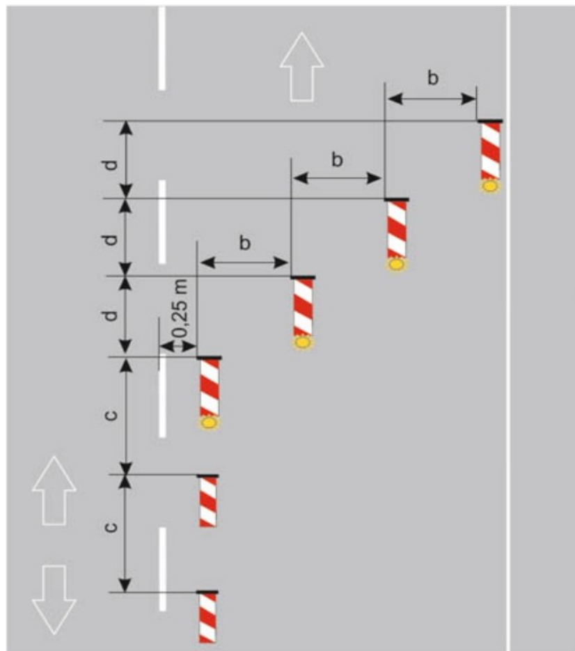
Slika 5. Raspored prometnih znakova i opreme u zoni početka suženja djela kolnika odnosno prometne trake
