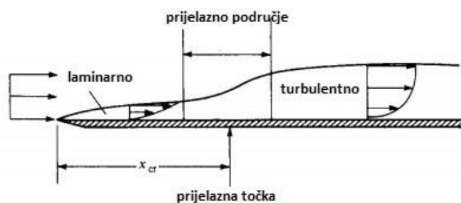
Slika 28. Prijelaz sa laminarnog u turbulentno strujanje, [1]
