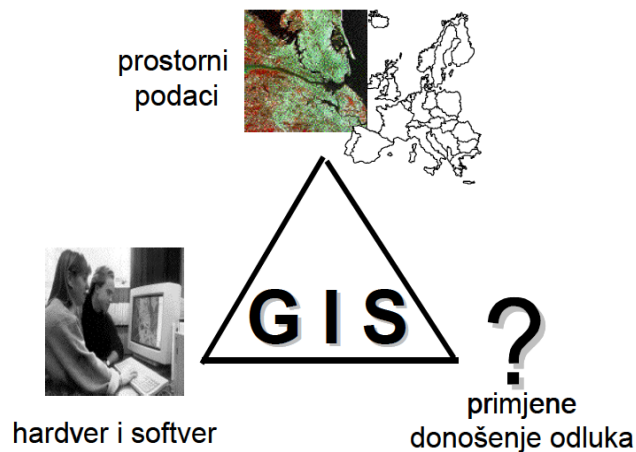
Slika 8. Komponente GIS-a
