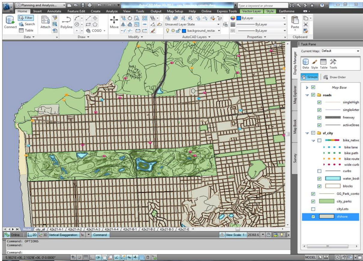
Slika 9. AutoCAD map
