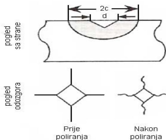
Slika 23. Medijan pukotina [7]
