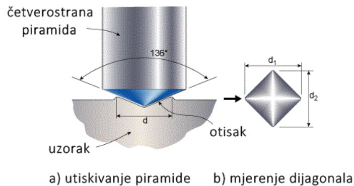
Slika 41. Vickersova metoda, [39]
