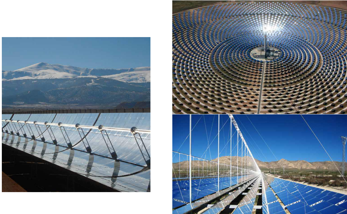
Slika 4. CSP tehnologije, Parabolična ogledala (lijevo), Solarni toranj (desno, gore), LRF (desno, dolje) [9]
