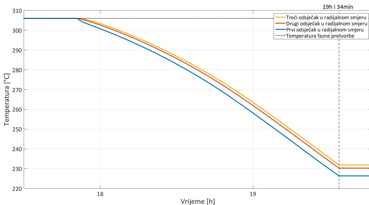
Slika 41. Detalj D – pražnjenje za medij u radijalnom smjeru za drugi odsječak u aksijalnom smjeru
