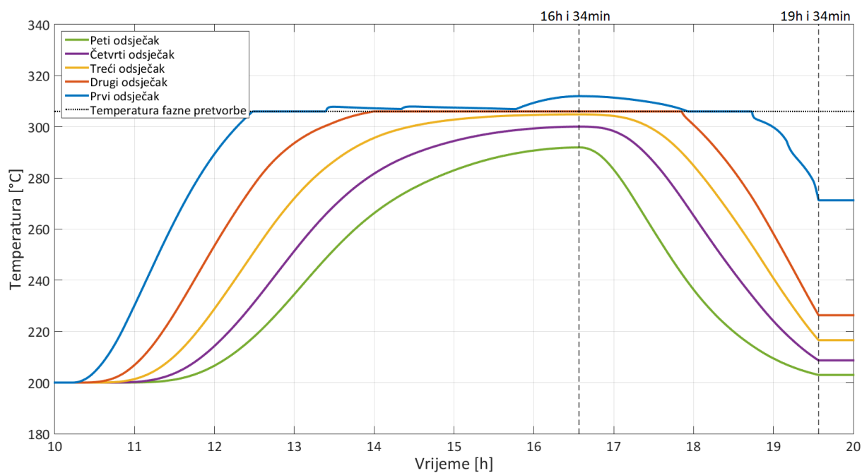
Slika 33. Temperaturni profil prvih odsječaka u radialnom smjeru, prikazani u aksijalnom smjeru
