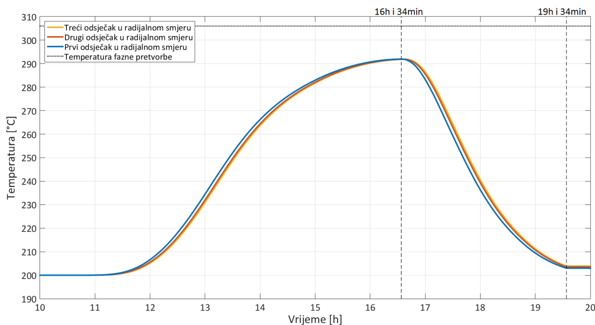
Slika 44. Temperaturni profil medija za pohranu toplinske energije u radialnom smjeru prikazan za peti odsječak u aksijalnom smjeru
