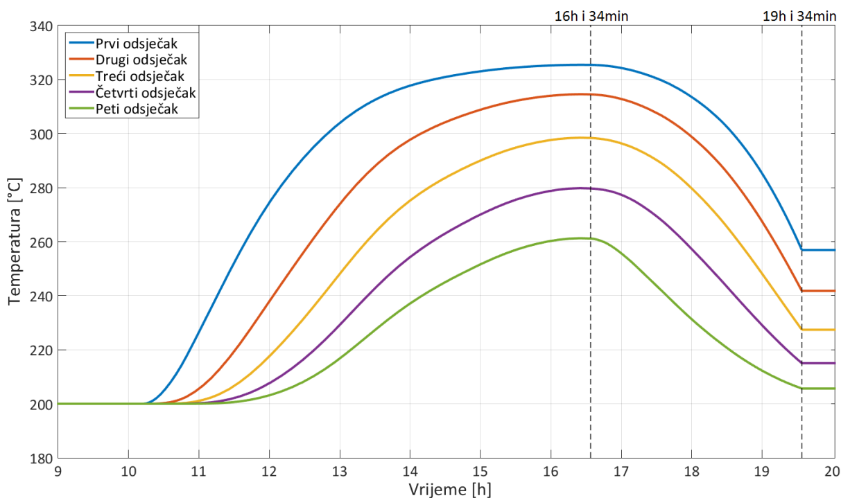
Slika 26. Temperaturni profil prvih odsječaka u radijalnom smjeru, prikazani u aksijalnom smjeru
