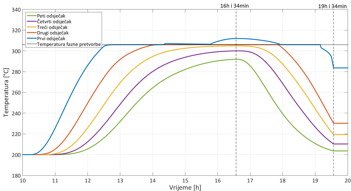
Slika 34. Temperaturni profil drugih odsječaka u radialnom smjeru, prikazani u aksijalnom smjeru
