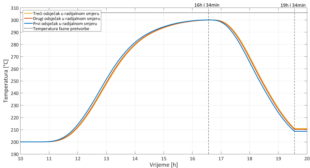
Slika 43. Temperaturni profil medija za pohranu toplinske energije u radialnom smjeru prikazan za četvrti odsječak u aksijalnom smjeru
