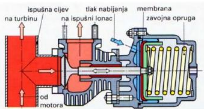
Slika 8. Regulacijski ventil turbopunjača [3]
