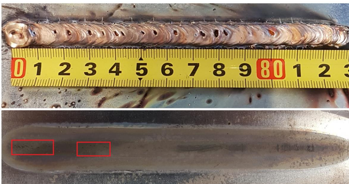
Slika 33. Uzorak 3B: - gornja slika: lice zalemljenog spoja - donja slika: naličje zalemljenog spoja
