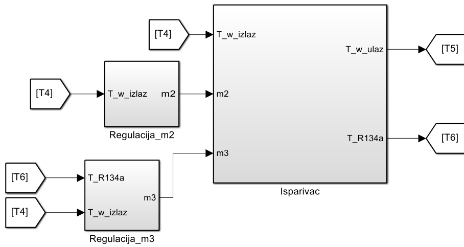
Shema 9 Isparivač
