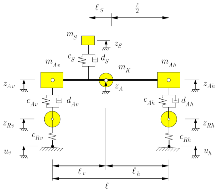
Slika 22. Shematski prikaz ravninskog modela vozila sa sjedalom (5 SSG) [5]
