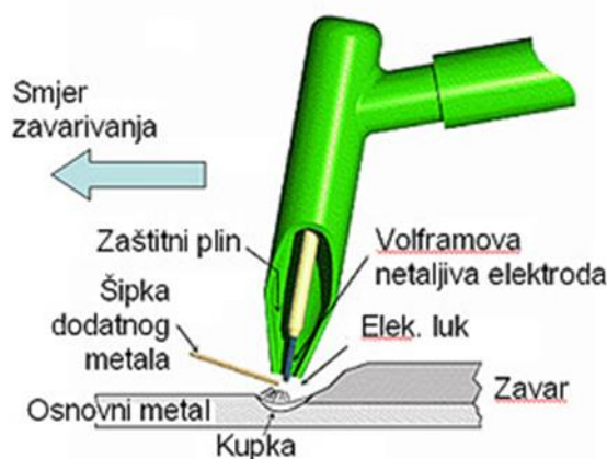
Slika 1. Shematski prikaz TIG postupka zavarivanja [4]
