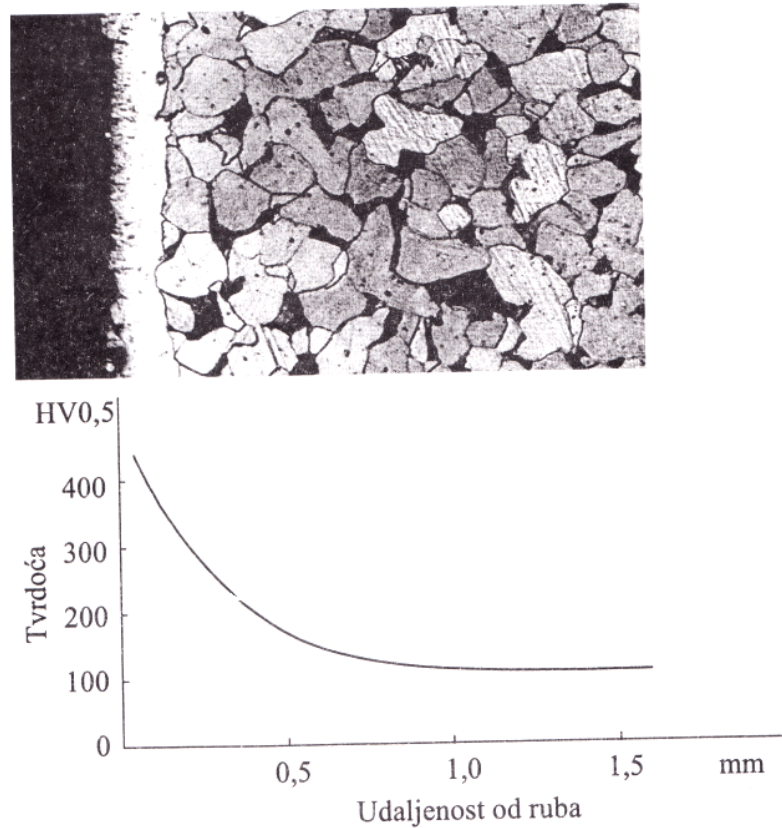
Slika 37: mikrostruktura i raspored tvrdoće poprečnog presjeka nitriranog elika [14]
