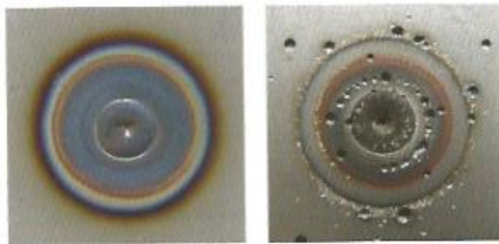
Slika 13. Utjecaj pobojanosti površine na pojavu pita nakon 24h ispitivanja u \text{FeCl}_3 [1]
