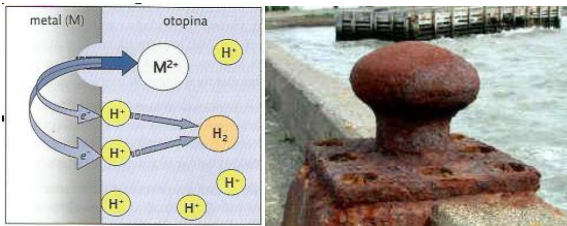
Slika 3. Shematski prikaz elektrokemijske korozije, i primjer opće korozije [1,5]
