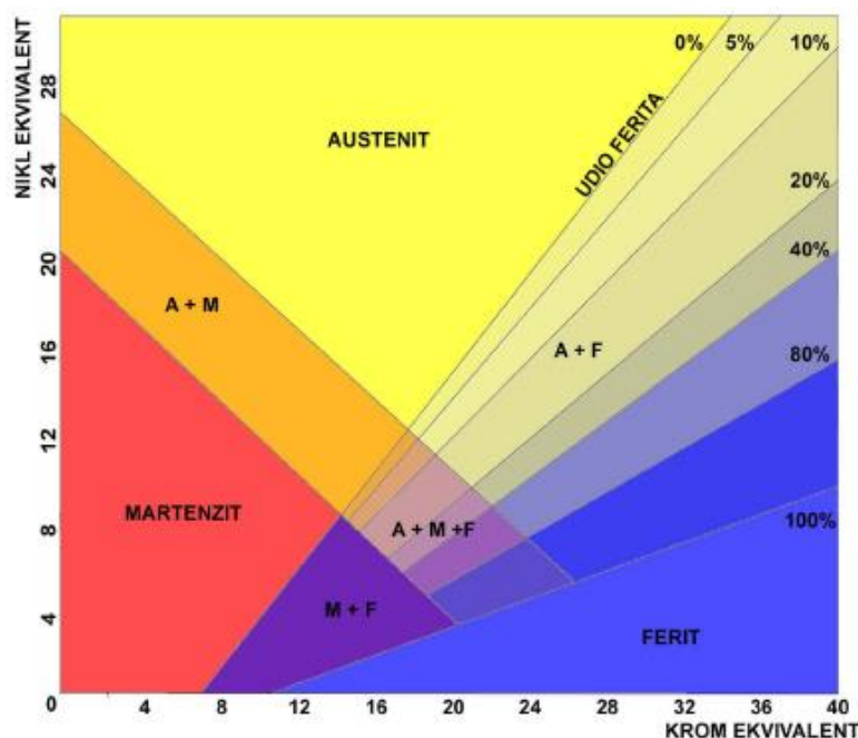
Slika 18. Schäfflerov dijagram struktura nehrđajućih čelika ovisno o udjelima Cr i Ni [10]
