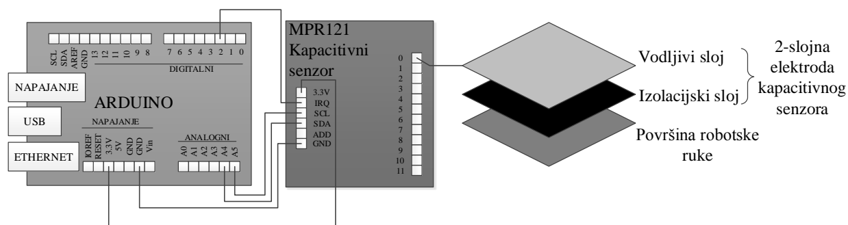
Slika 3.2. Kapacitivni senzor.
