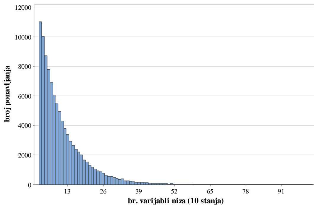
Slika 4.14. Razdioba dužine lanaca za deset stanja.
