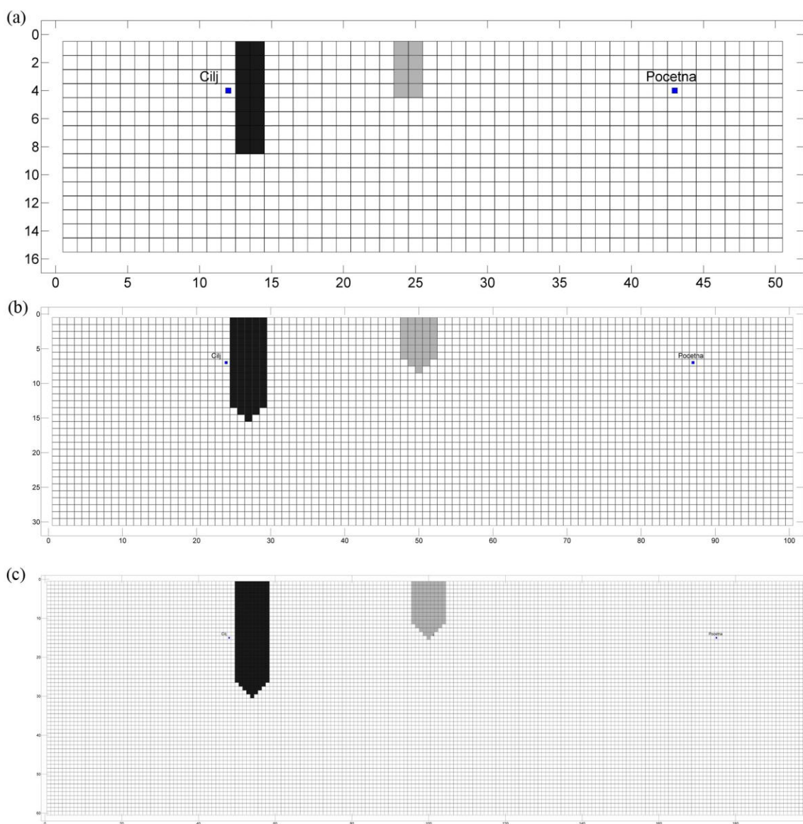
Slika 3.21. Diskretizacija prostora: a) 15 x 50, b) 30 x 100, c) 60 x 200.
