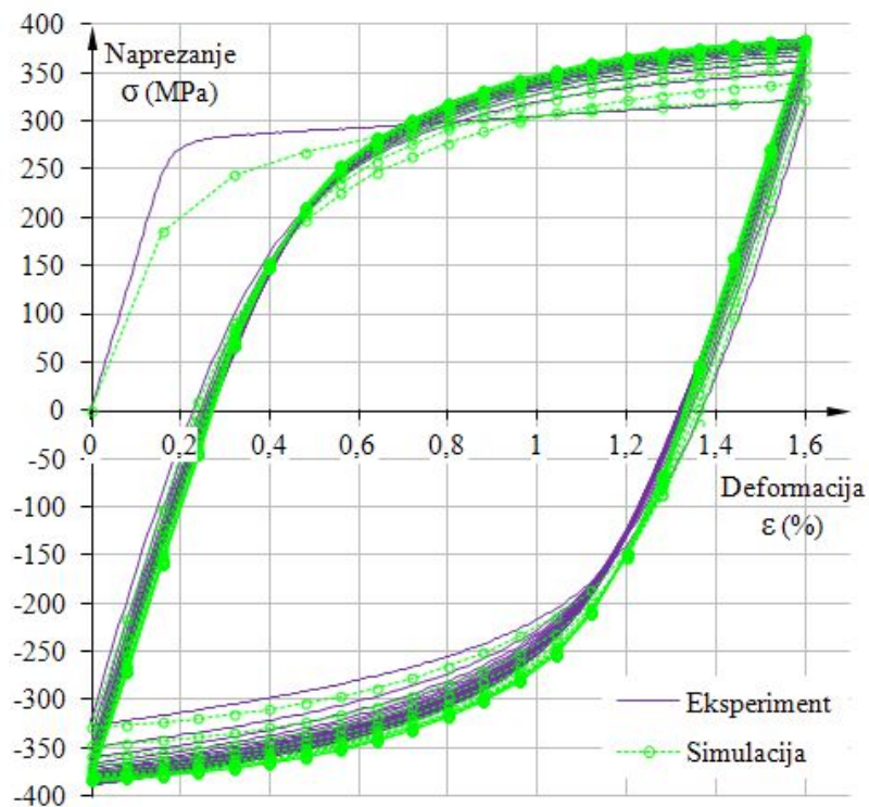
Slika 94. Usporedba asimetričnog ispitivanja i rezultata numeričke analize za \epsilon_{min/max}=0/+1,6 % (Nestand.)
