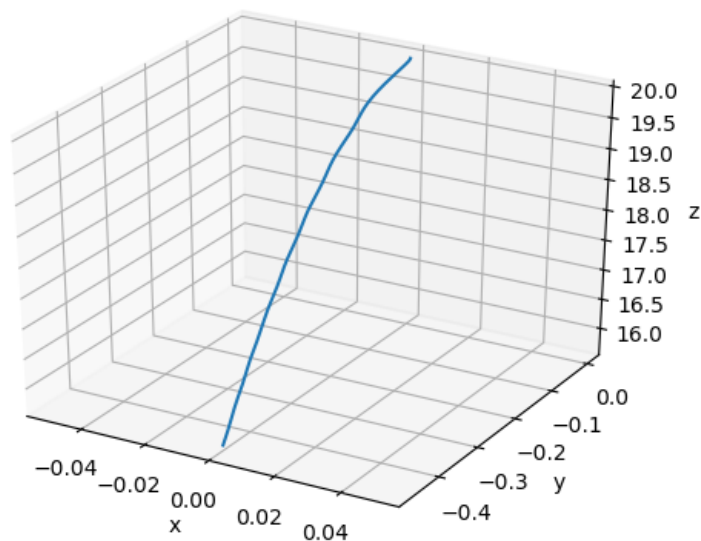
Slika 7: Trajektorija letjelice
