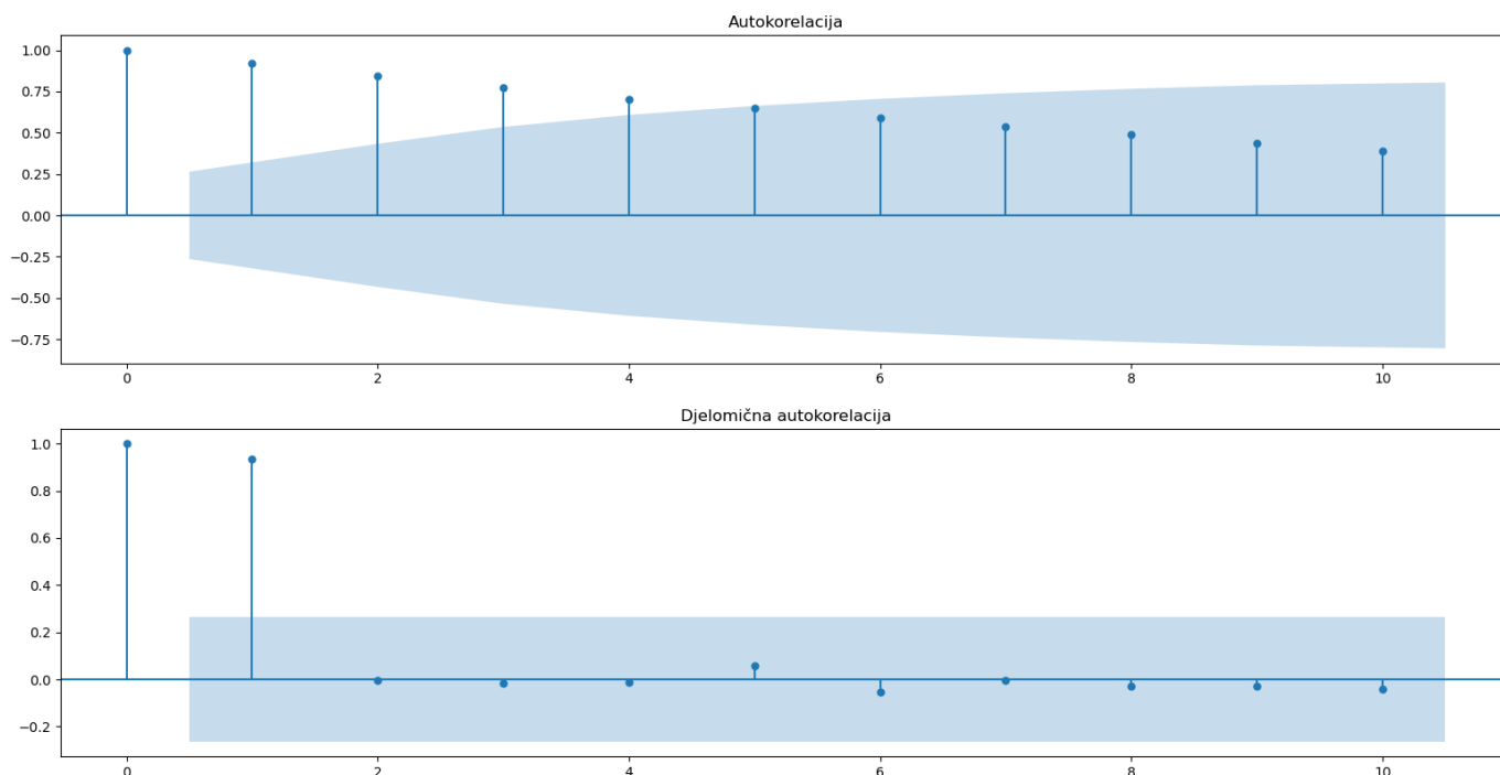
Slika 16. ACF i PACF dijagram za potvrđene slučajeve
