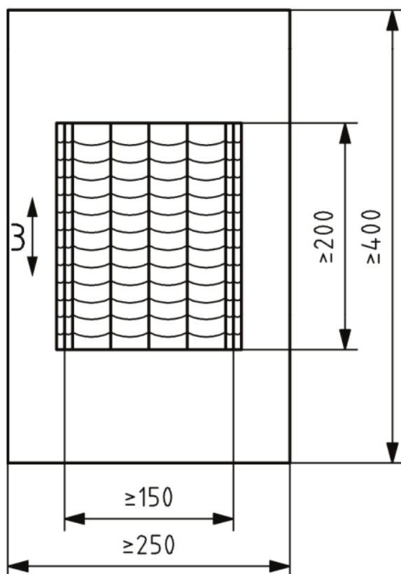
Slika 9 pločasti ispitni uzorak za navarivanje [10]
