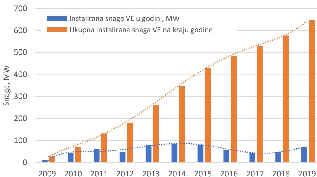
Slika 4.1: Instalirana snaga vjetroelektrana u RH [9]
