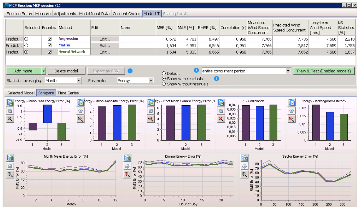
Slika 7.21: Usporedba MCP matematičkih modela za predviđanje [28]
