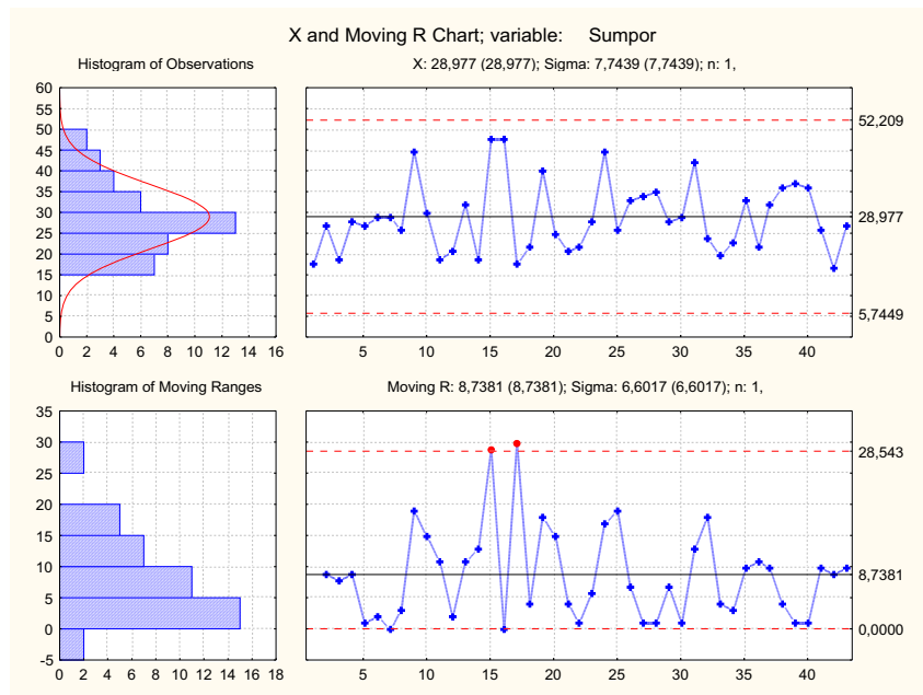
Slika 80. \bar{x} -MR kontrolna karta vrijednosti mjerenja količine ukupnog sumpora
