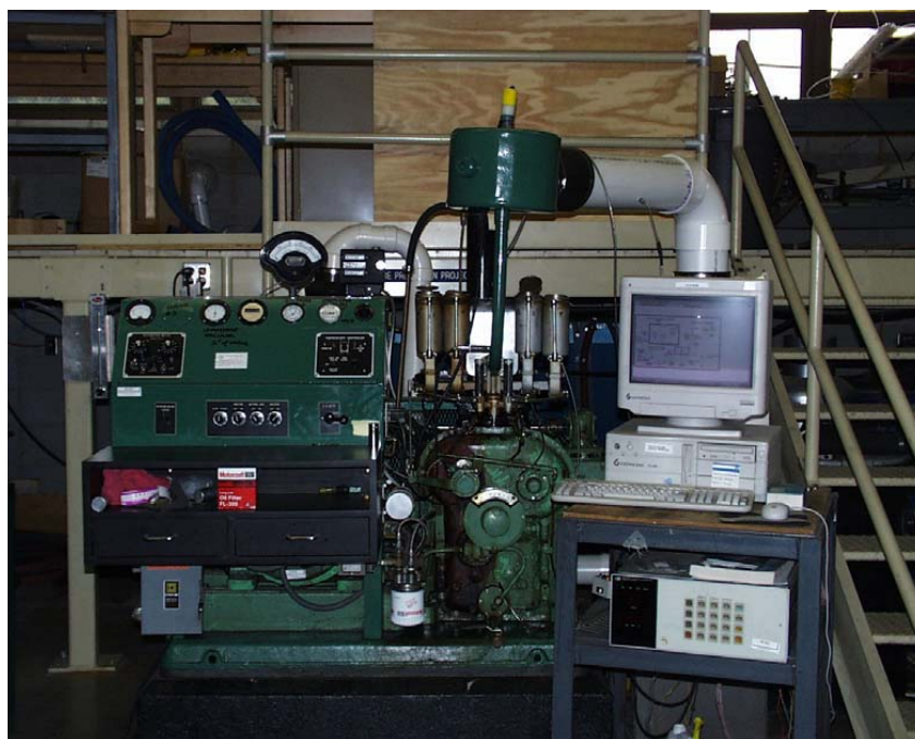
Slika 82. Aparatura za određivanje IOB-a
