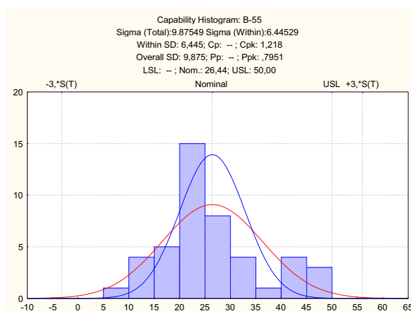
Slika 40. Histogram vrijednosti mjerenja količine ukupnog sumpora za spremnik B-55
