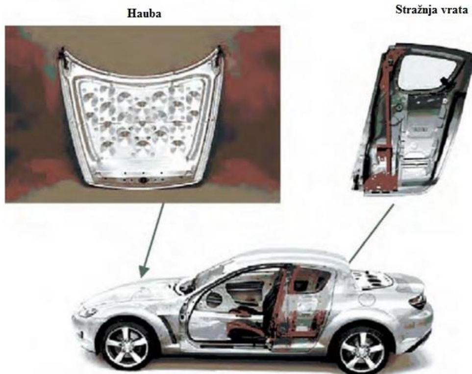
Slika 34 Primjena zavarivanja aluminijskih dijelova trenjem na Mazda RX-8 automobilu [3]
