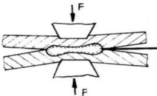
Slika 5 Istiskivanje [9]
