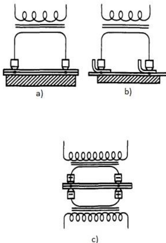
Slika 11 Serijsko zavarivanje [8]
