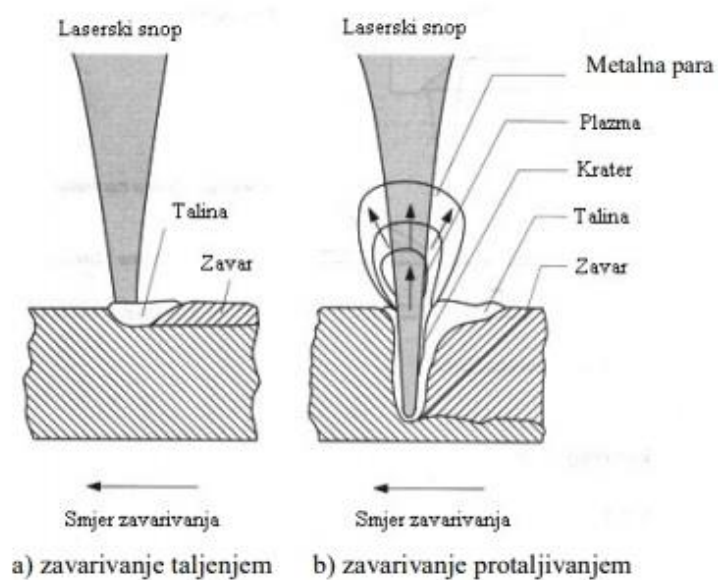
Slika 28 Tehnike zavarivanja laserom [23]
