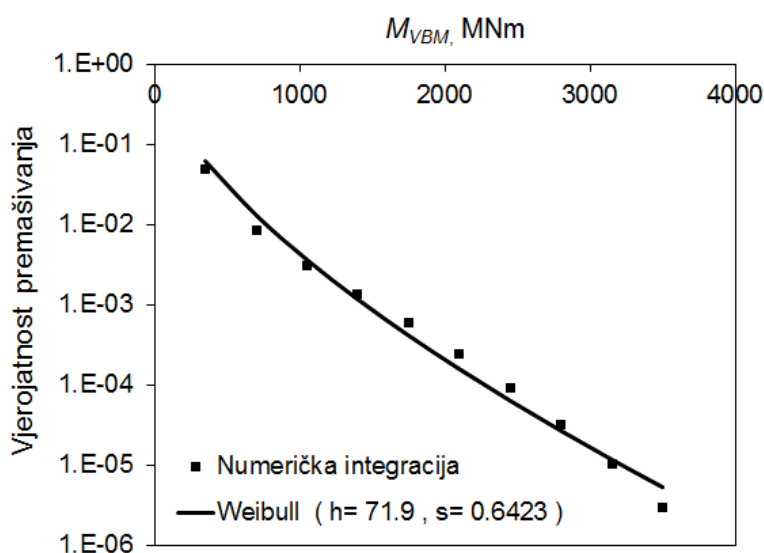
Slika 3.8. Raspodjela vjerojatnosti premašivanja vertikalnog valnog momenta savijanja, tipično sudarno okruženje [87]
