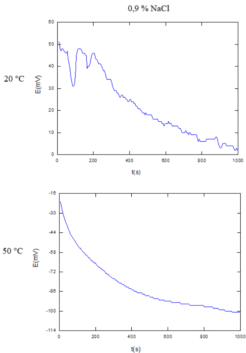
Slika 42. Dijagrami određivanja korozivnog potencijala za čelik 316L
