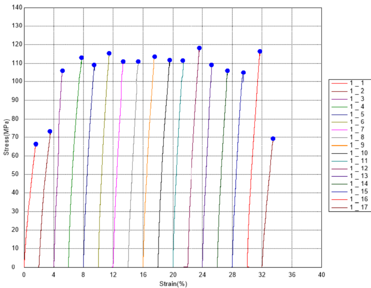
Slika 10. Dijagram naprežanje-istežanje za UP/4lan
