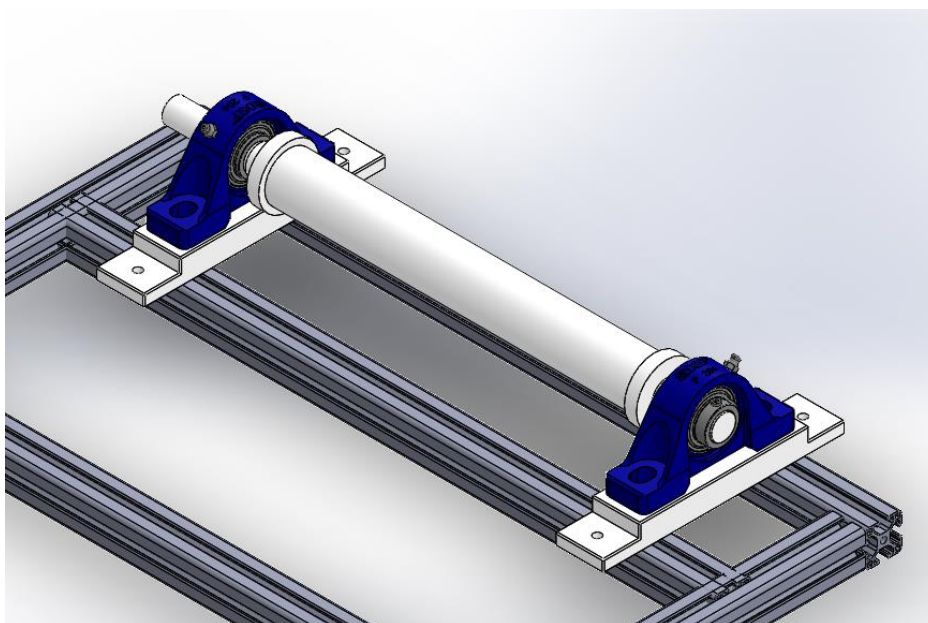
Slika 3.5 Spoj vratila i kućišta na postolja
