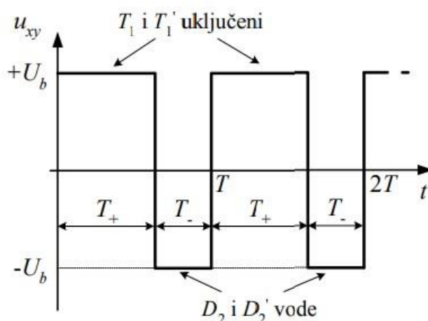
Slika 4.8 PWM signal [11]
