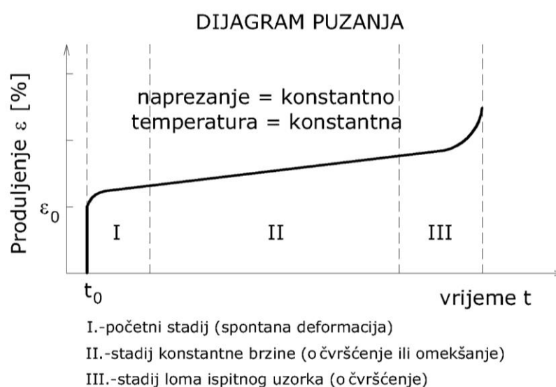
Slika 7. Dijagram puzanja [5]
